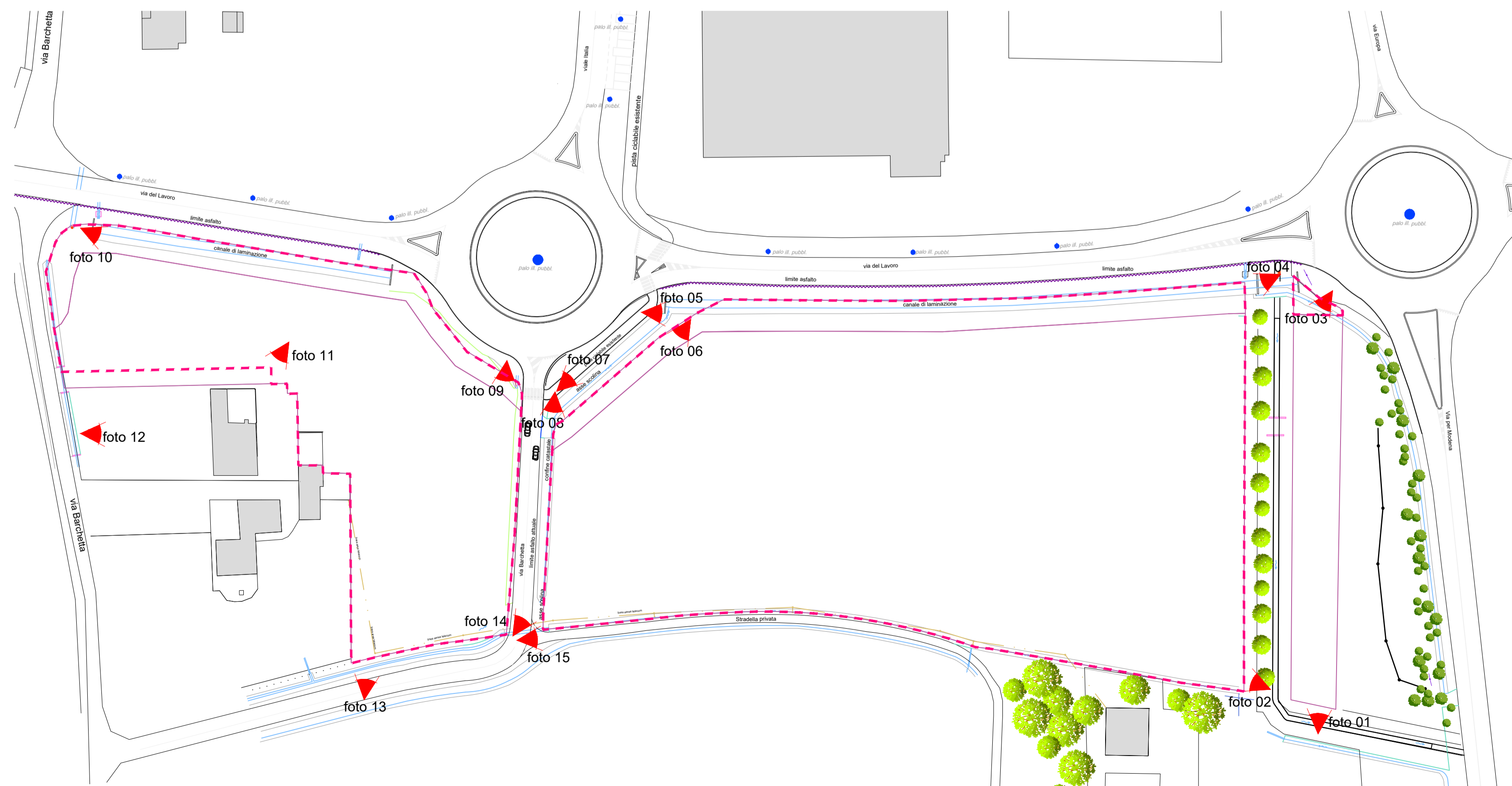
PLANIMETRIA GENERALE - Stato attuale scala 1:1000
