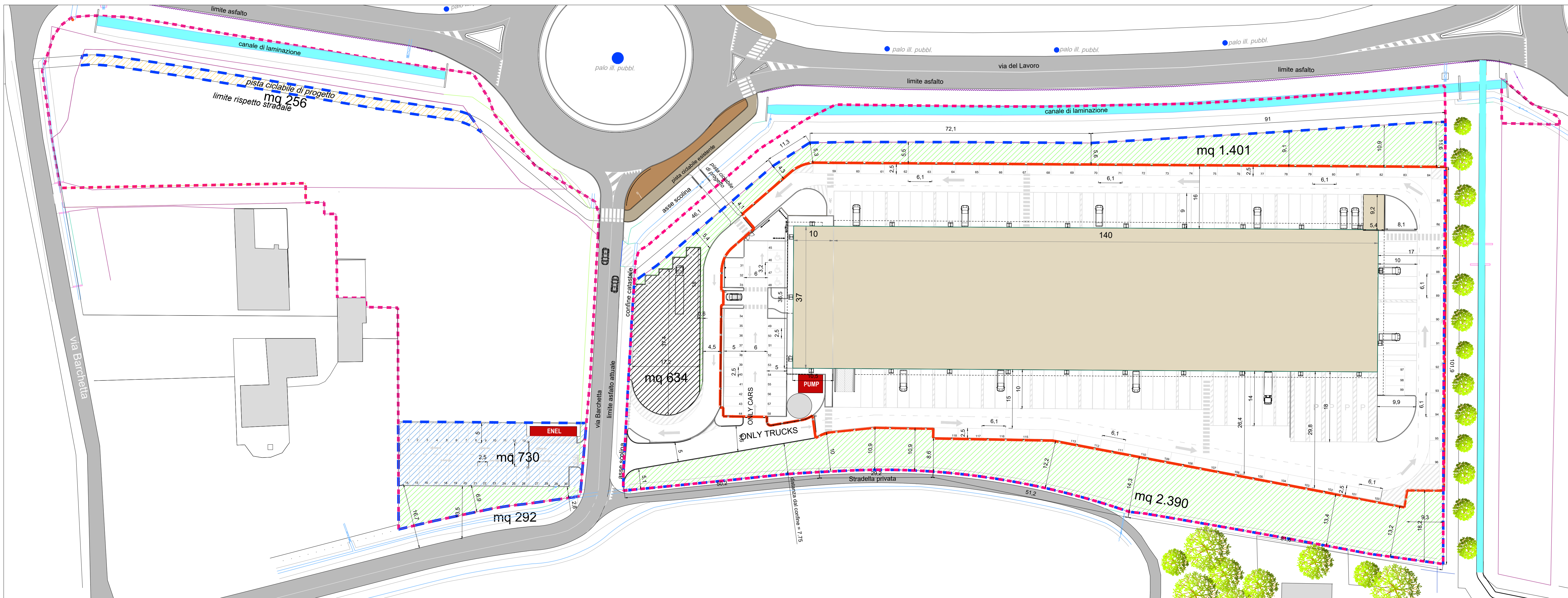
DOTAZIONI IN CESSIONE scala 1:1000
