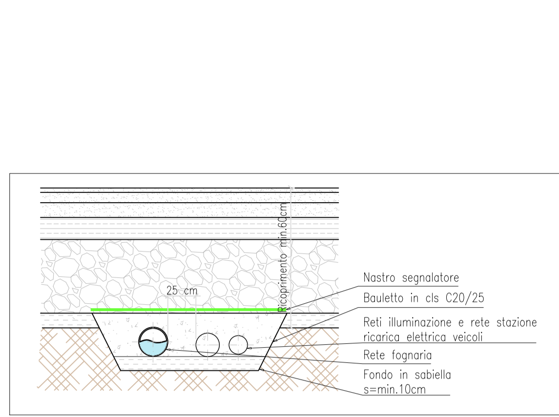
DETTAGLIO TIPO Bauletto in cls reti fognarie+illuminazione SCALA 1:25
