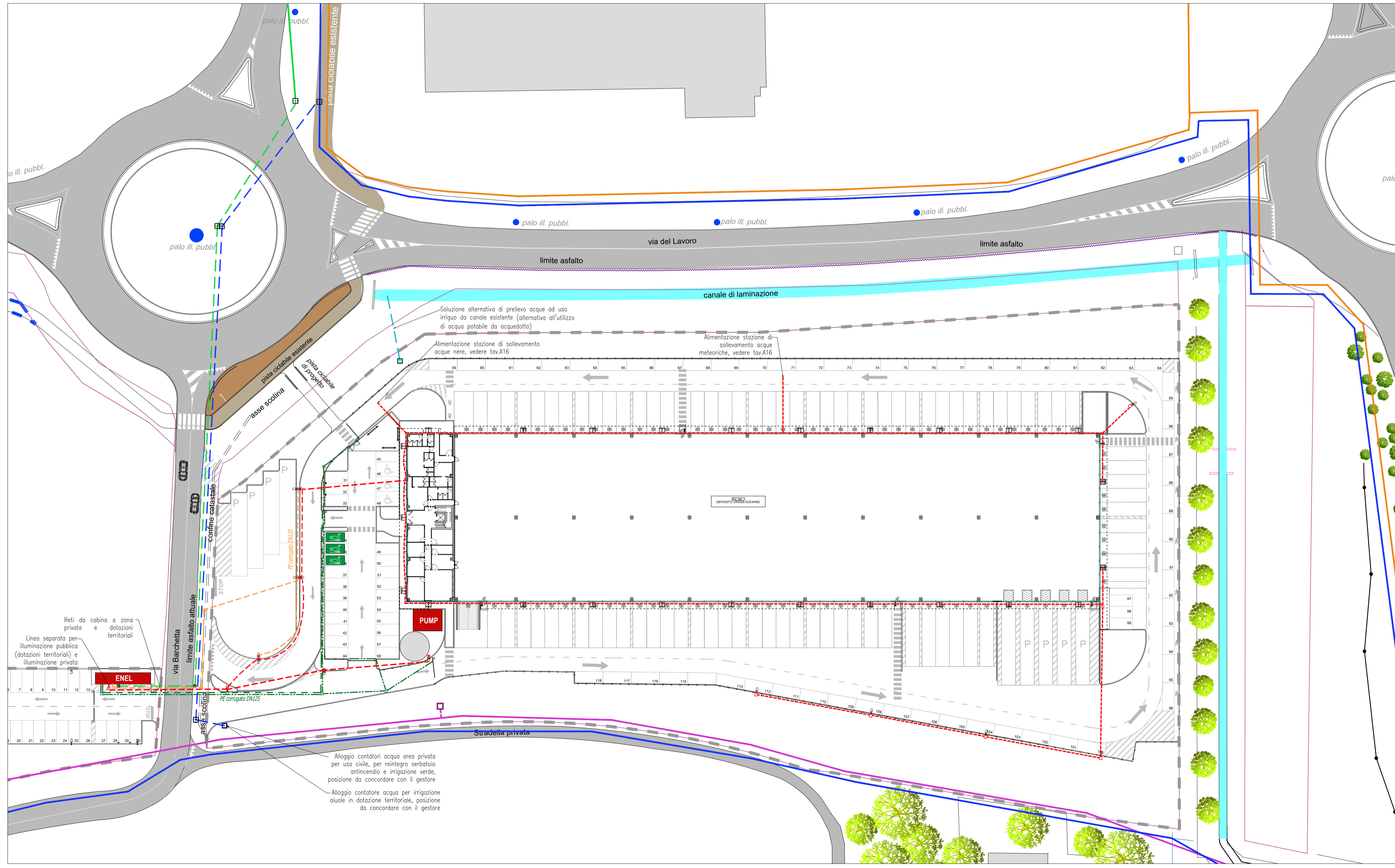
SCHEMA RETI E UTENZE SCALA 1:500
