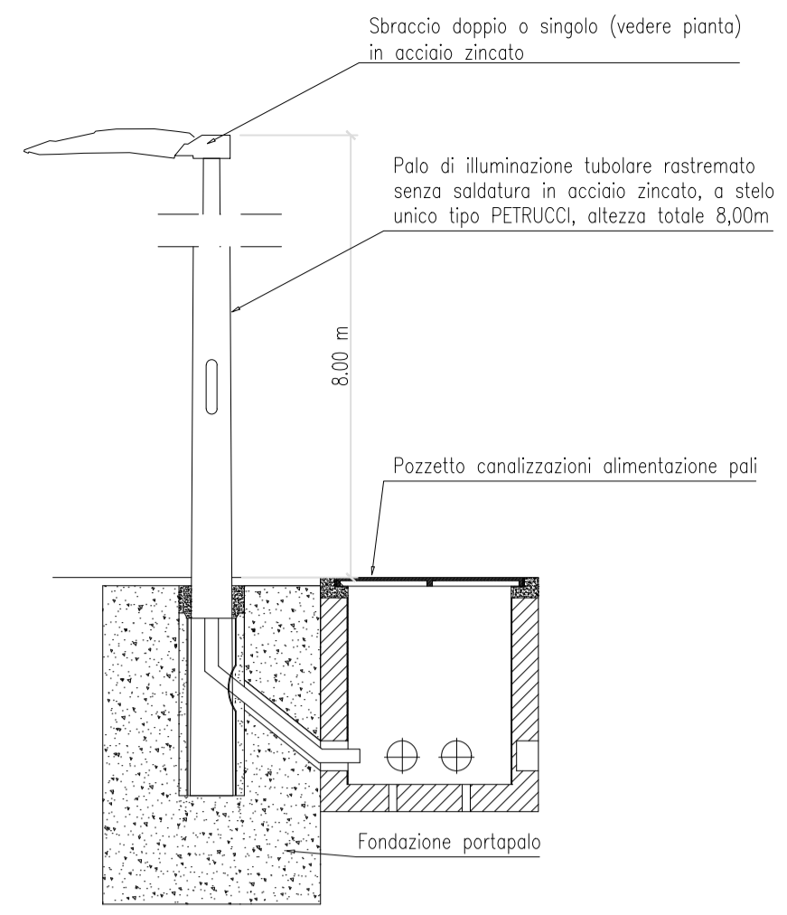
DETTAGLIO TIPO Palo Illuminazione SCALA 1:50
