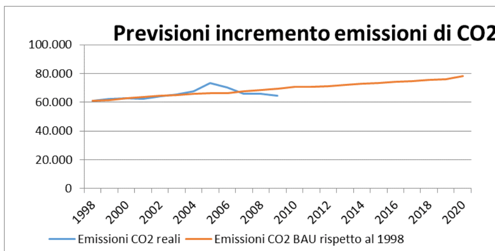
Figura 10 - Previsione al 2020 delle emissioni di CO 2 (t) in base alle previsioni demografiche
